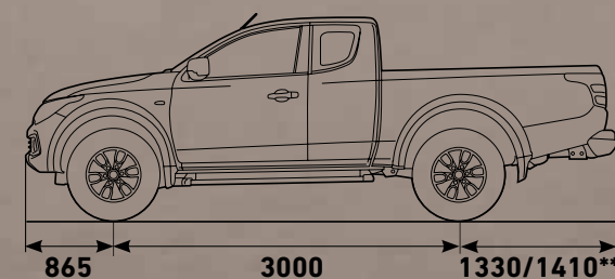
VERZE EXTENDED CAB (PRODLOUŽENÁ KABINA - 4 SEDADLA)
